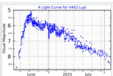
Curva de luz de banda visual para V462 Lupi, trazada a partir de datos de AAVSO [5] y ASAS-SN [1] (punto rojo)
