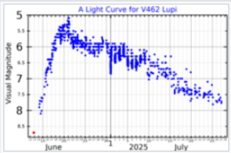
Eine visuelle Bandlichtkurve für V462 Lupi, erstellt aus Daten von AAVSO [5] und ASAS-SN [1] (roter Punkt)
